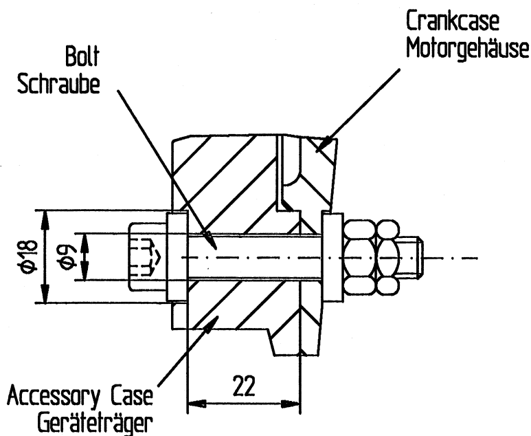
Abb. 1 Geräteträgerbefestigung (Ausschnitt)
